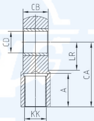
内螺纹活塞杆单耳环外形及连接尺寸
