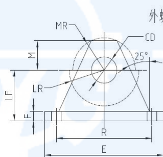
外螺纹活塞杆耳环（关节轴承）用耳环架外形及连接尺寸
