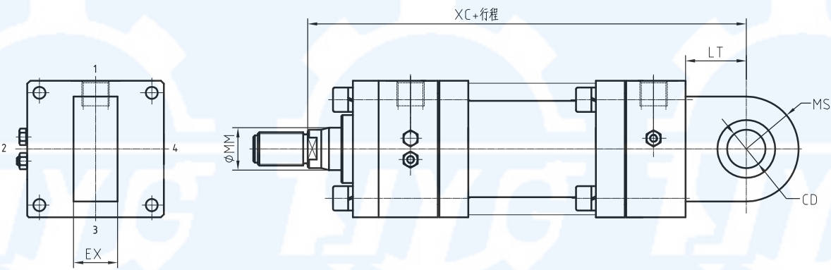
缸底单耳环带关节轴承油缸 MP5
