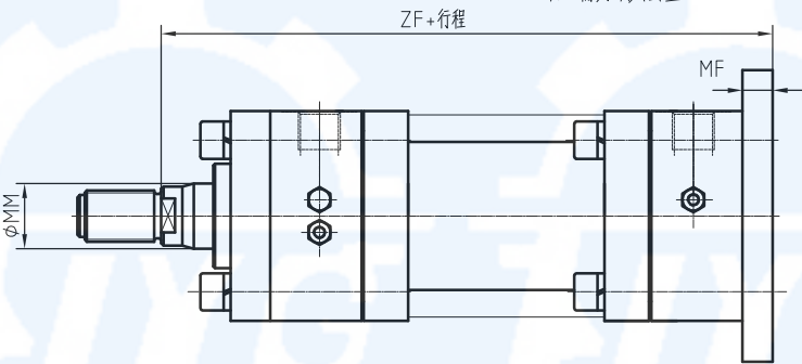
后端方形法兰 MF6
