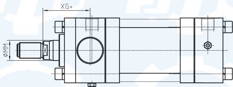
前铰轴型油缸 MT1
