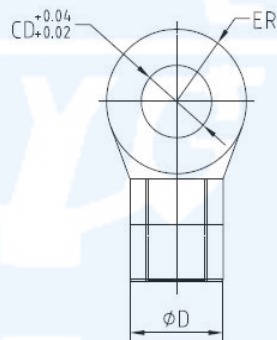
内螺纹活塞杆双耳环外形及连接尺寸
