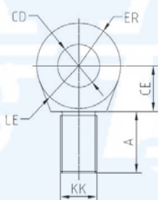
外螺纹活塞杆耳环（关节轴承）外形及连接尺寸
