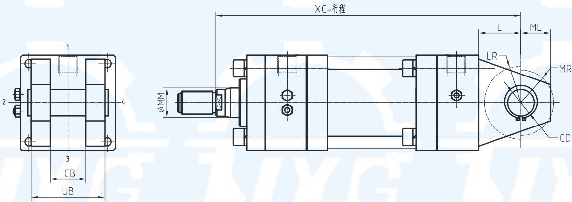
缸底双耳环油缸 MP1
