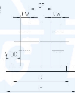
外螺纹活塞杆耳环（关节轴承）用耳环架
