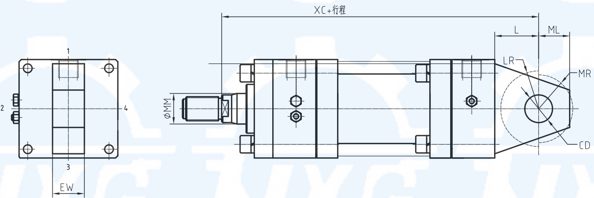
缸底单耳环油缸 MP3
