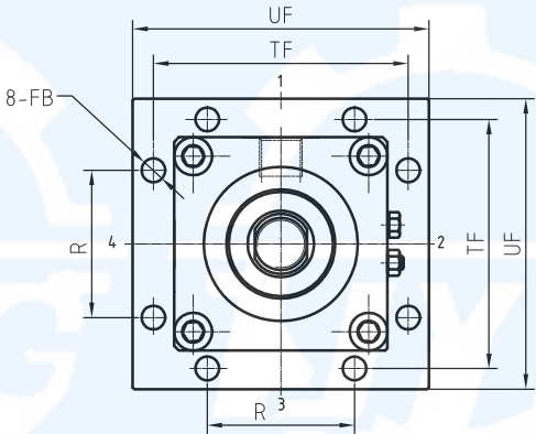
后端方形法兰 MF6
