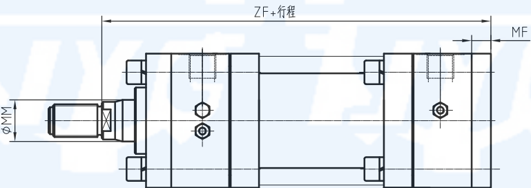
后端矩形法兰 MF2
