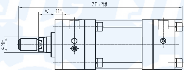
前端矩形法兰 MF1
